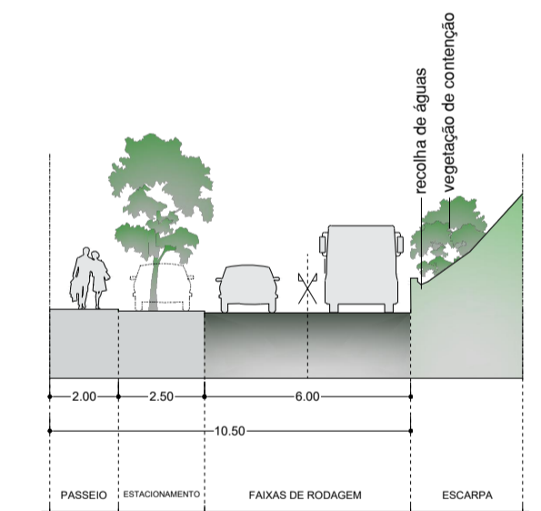
PERFIS TIPO: ESC. 1/200
